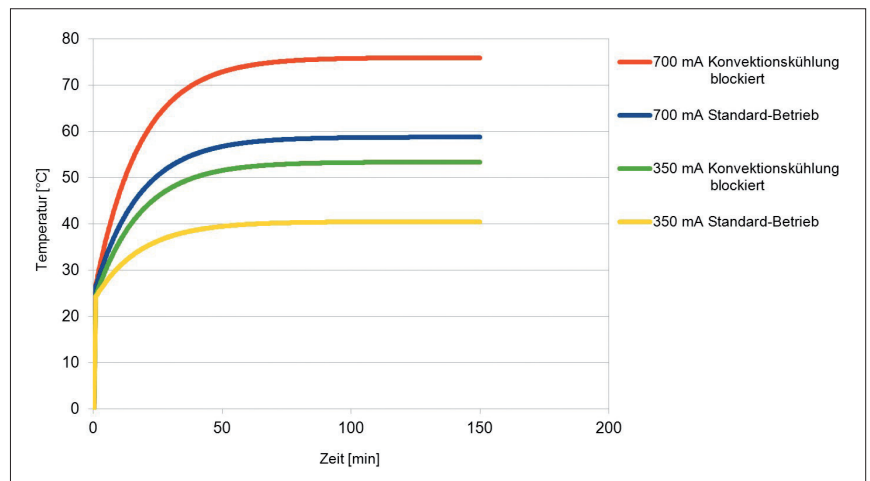
Temperaturkurven Leuchtenkörper (60 LEDs, Umgebungstemperatur 25°C)
