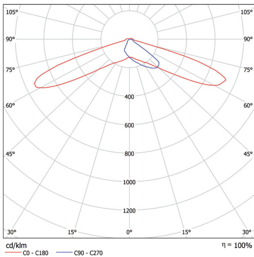
Lichtstärkeverteilungskurve (LVK) Eulumdaten auf Anfrage
